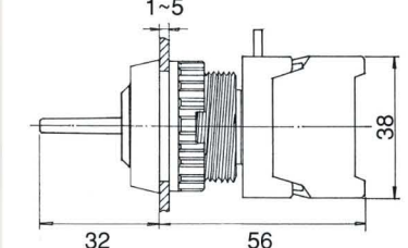
LUS30-2/O , 1→0←2 , Spring return LUS30-2/C , 1→0←2 , Spring return
